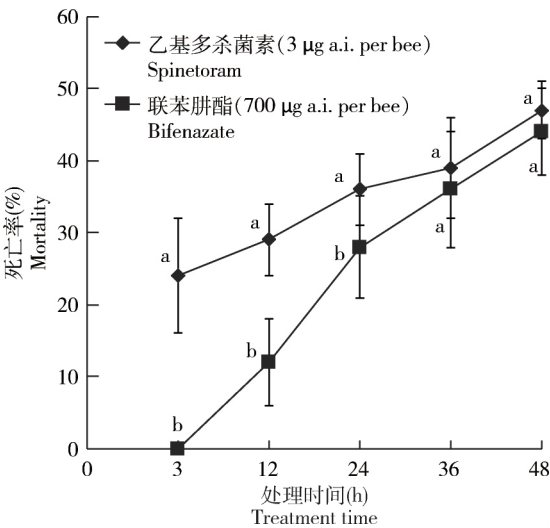
图 1 致死中剂量的乙基多杀菌素和联苯肼酯处理不同时间后地熊蜂采集蜂的死亡率
