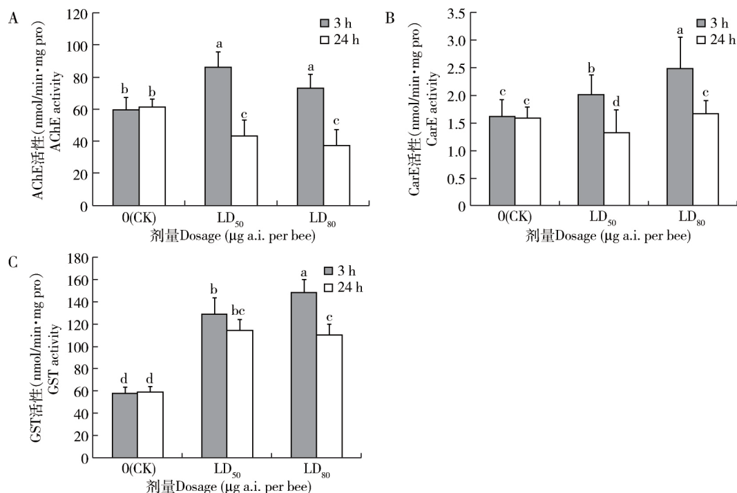
图 2 乙基多杀菌素对地熊蜂成年工蜂头部乙酰胆碱酯酶 (A)、腹部羧酸酯酶 (B) 和谷胱甘肽-S-转移酶 (C) 活性的影响
