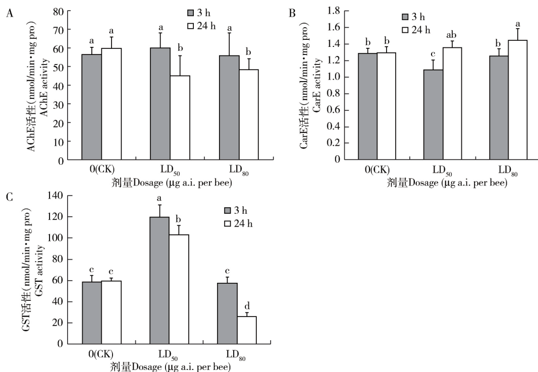
图3 联苯肼酯对地熊蜂成年工蜂头部乙酰胆碱酯酶 (A)、腹部羧酸酯酶 (B) 和谷胱甘肽-S-转移酶 (C) 活性的影响
